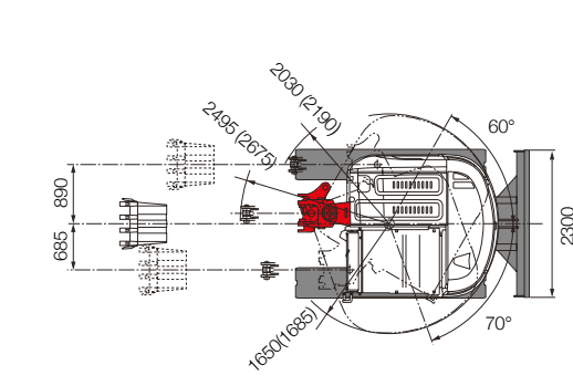
Mono Boom
