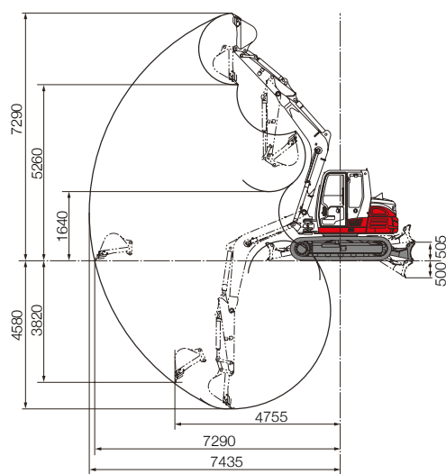
Mono Boom
